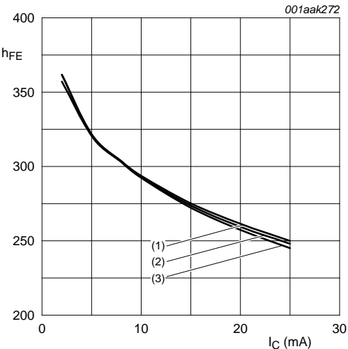
T amb = 25 °C. (1) V CE = 1 V (2) V CE = 1.5 V (3) V CE = 2 V
