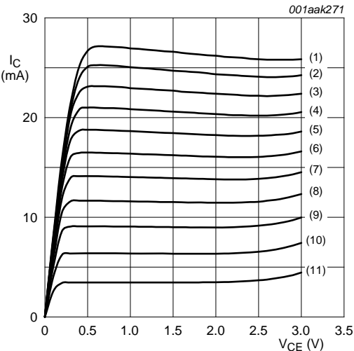
T amb = 25 °C. (1) I B = 110 μA (2) I B = 100 μA (3) I B = 90 μA (4) I B = 80 μA (5) I B = 70 μA (6) I B = 60 μA (7) I B = 50 μA (8) I B = 40 μA (9) I B = 30 μA (10) I B = 20 μA (11) I B = 10 μA
