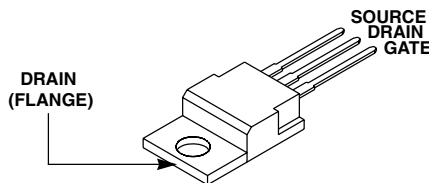
JEDEC TO-220AB
