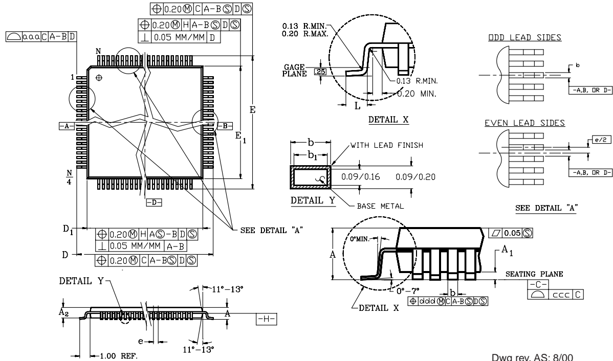
LQFP 064
