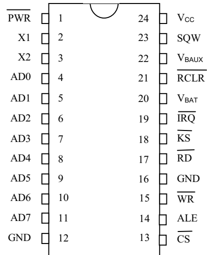
DS1685 24-Pin DIP DS1685S 24-Pin SOIC DS1685E 24-Pin TSSOP
